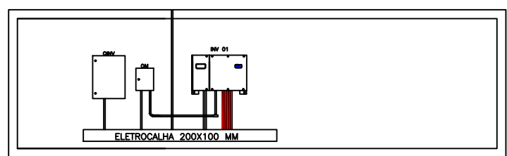
VISTA FRONTAL DOS INVERSORES E QUADROS
